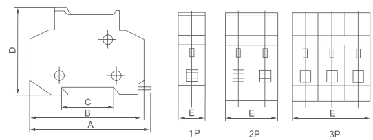
Dimensiones bases
